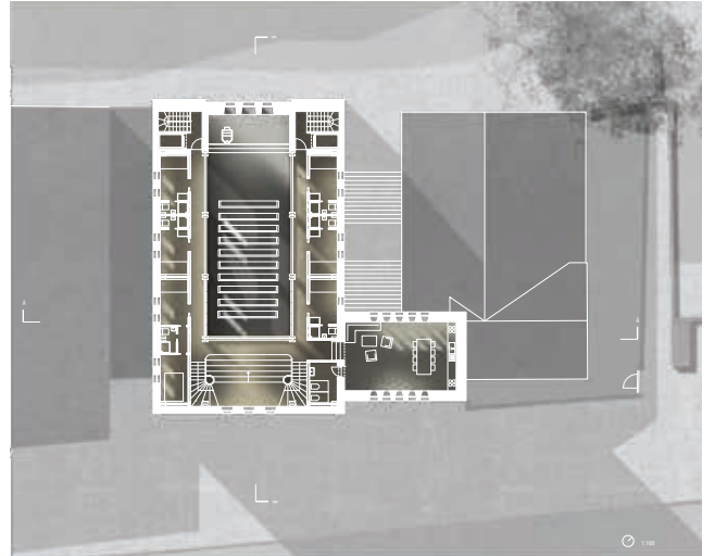
plan 7' étage, village de Valentin
